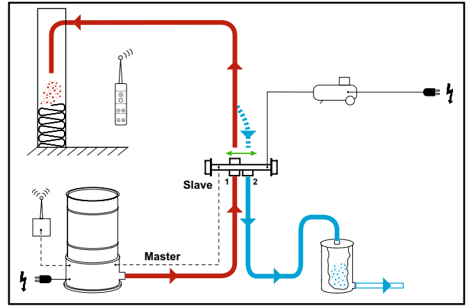
Drucklosschaltung
