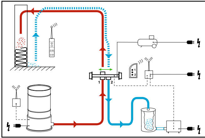
Einblasen und Absaugen
