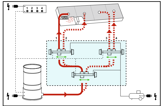
Stationäre Elementbefüllung im Werk
