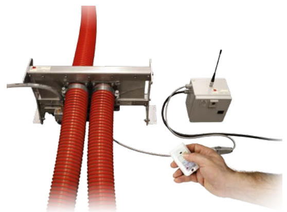
Einsatzbereite Flockenweiche mit Funkfernsteuerung
