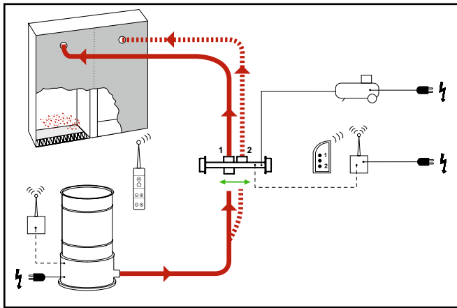
Einblasen mit zwei Schläuchen bzw. Vorschläuchen
