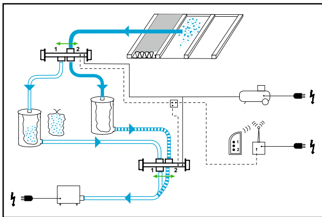
Unterbrechungsfreies Absaugen
