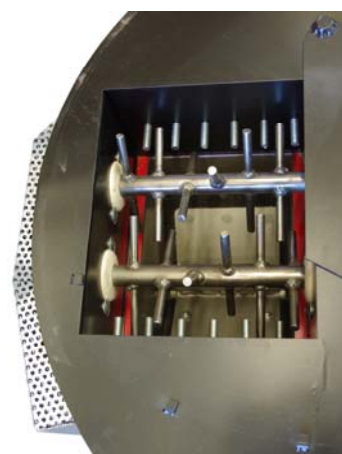
Nahaufnahme Häckselwellen
